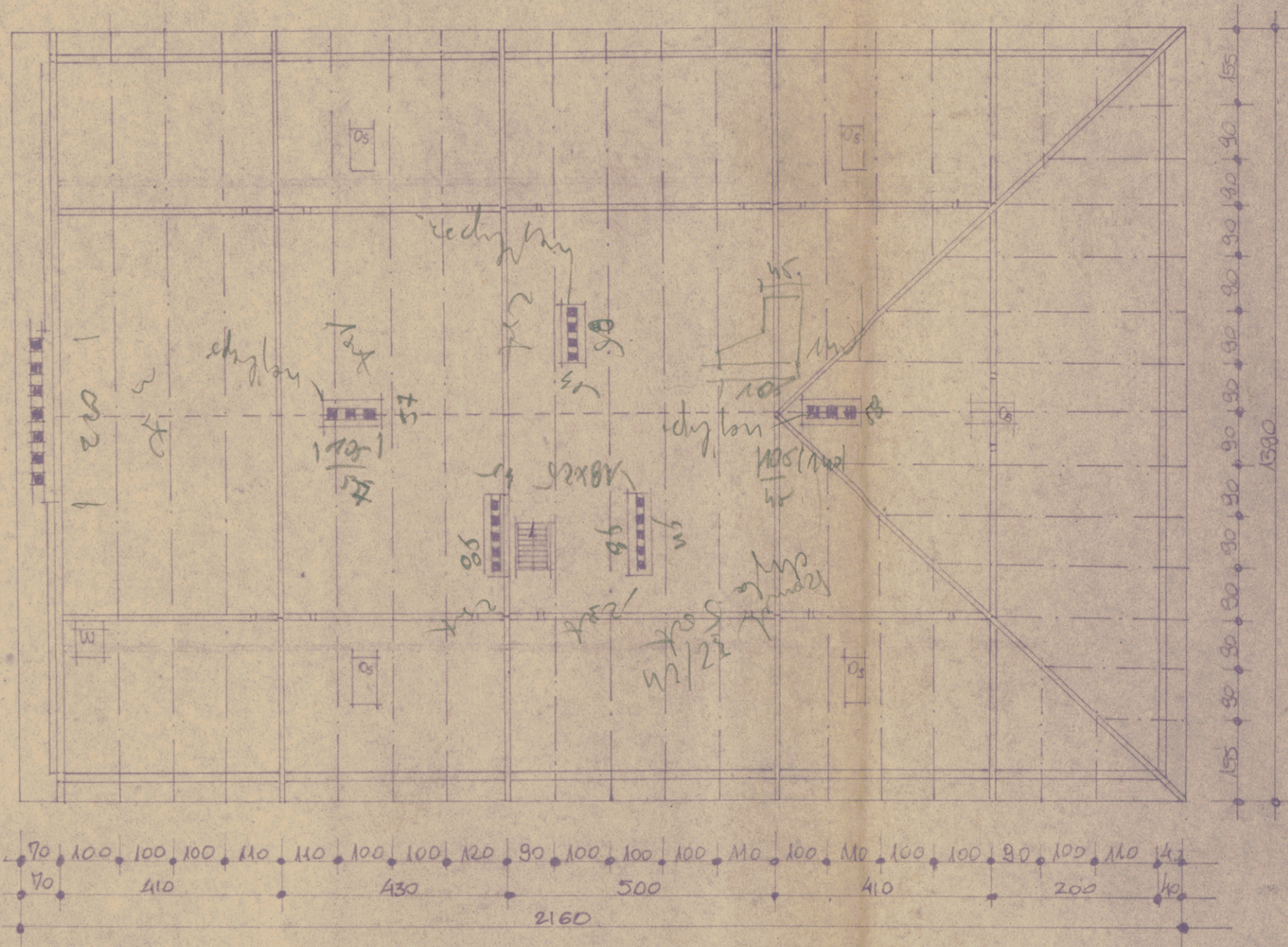
RZUT WIĘZBY DACHOWEJ SKALA 1:100
